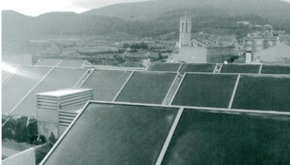
Imatge del 2010 de les instal·lacions d'energia tèrmica de l'edifici de les oficines d'Electra Caldense
