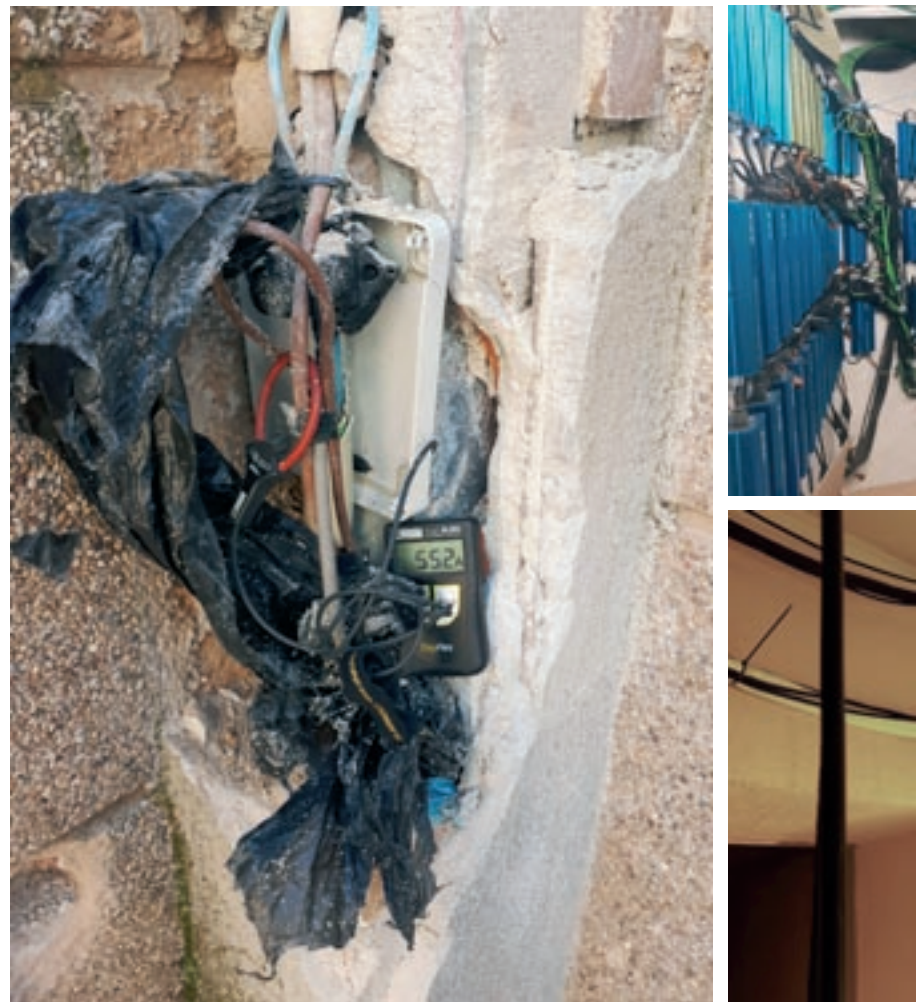
Exemples d'instal·lacions elèctriques manipulades detectades per Endesa en diversos punts del
