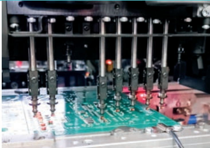
Línia de producció de plaques electròniques de Montronic
